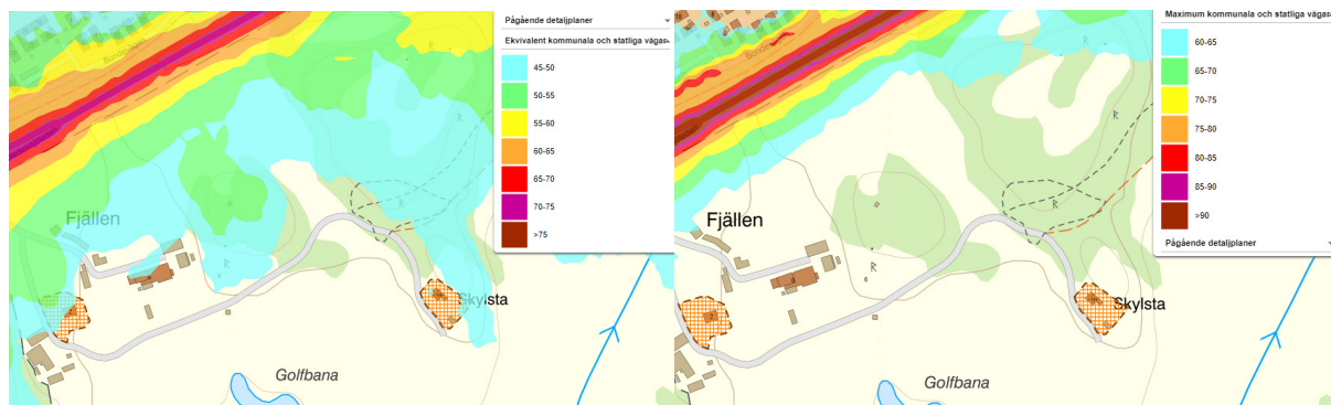
Figur 14: Ekvivalenta bullernivåer
